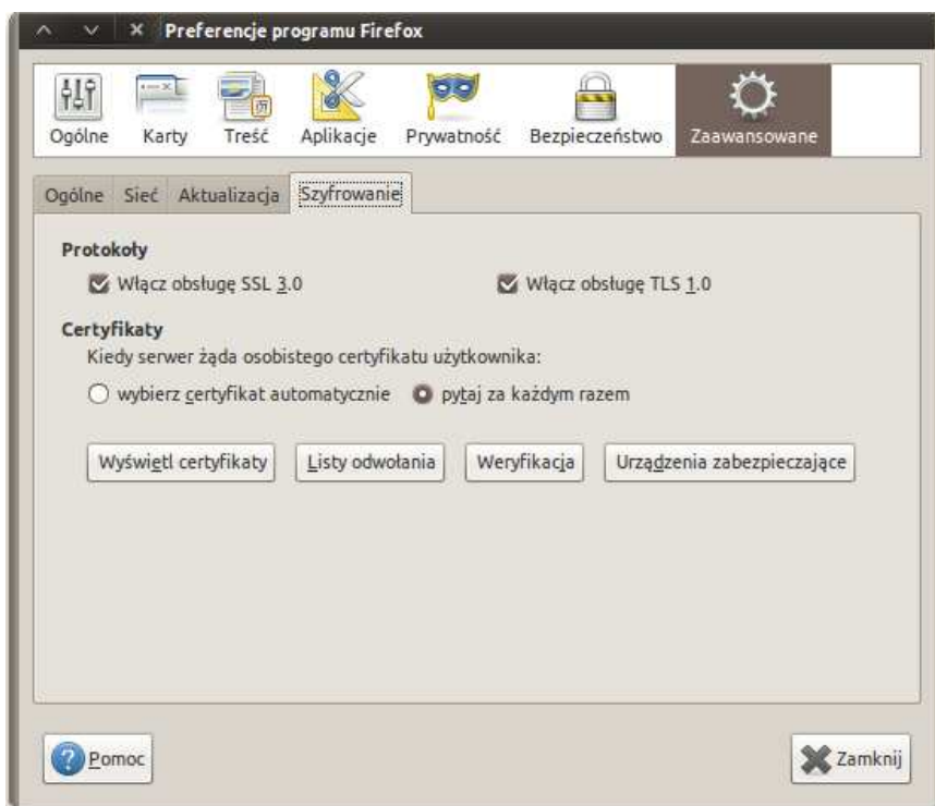
Rys.4. W zakładce Zaawansowane → Szyfrowanie możemy sprawdzić, czy na pewno mamy uruchomioną opcję obsługi protokołów SSL i TLS oraz ustawić dodatkową opcję pytania nas za każdym razem, gdy serwer wymaga certyfikatu użytkownika.
