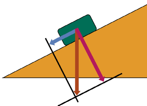
Rys. 12. Równia pochyła – schemat rozkładu sił
